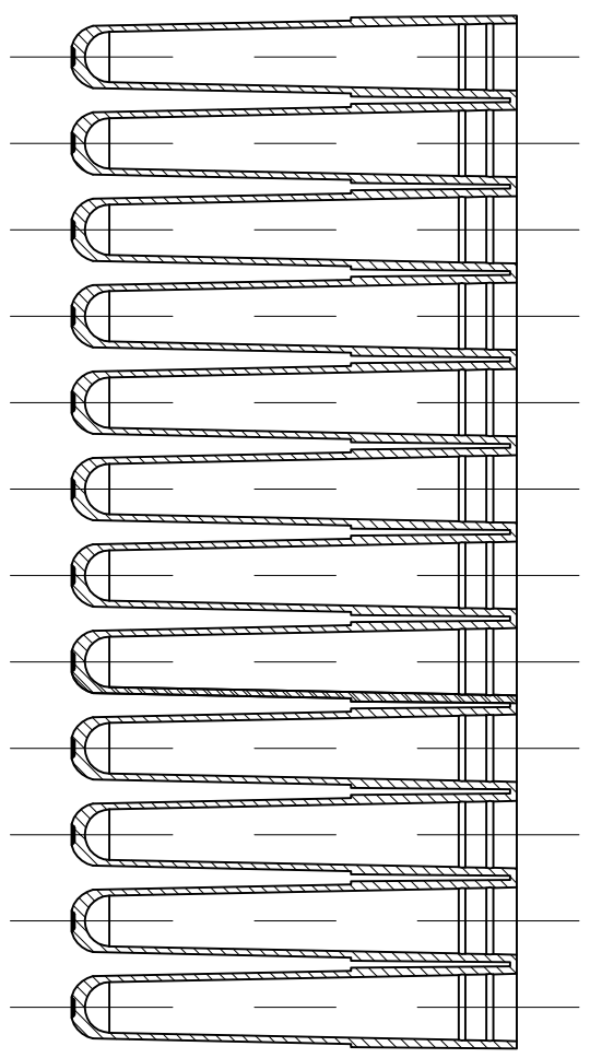
SECTION A-A
